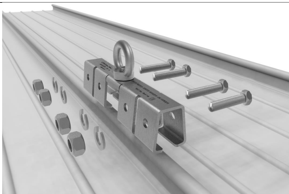
Schema di fissaggio AGGR-1A
