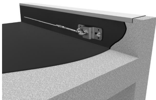
Fissaggio con barre filettate e ancorante chimico
