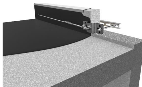
Fissaggio con barre filettate passanti nel supporto e contro piastra
