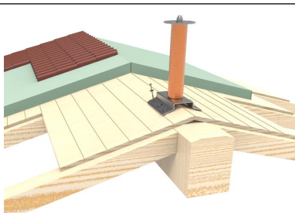
Fissaggio con viti legno
