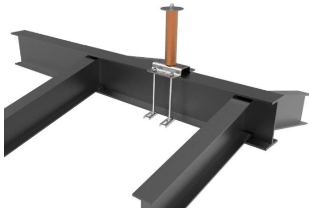
Incravattamento del supporto
