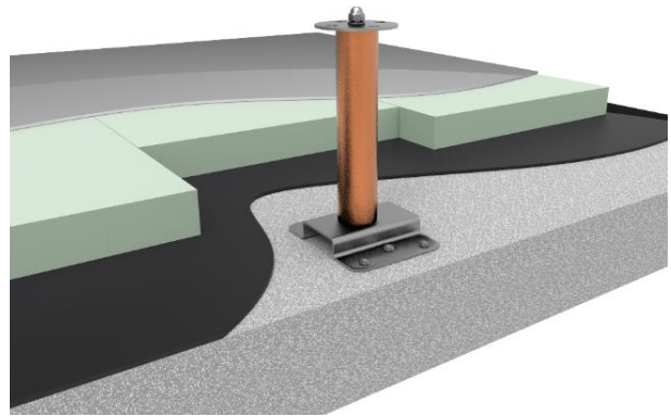
Fissaggio con viti cemento
