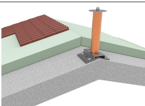
Fissaggio con barre filettate e ancorante chimico
