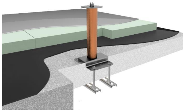
Barre filetate passanti e contropiastra
