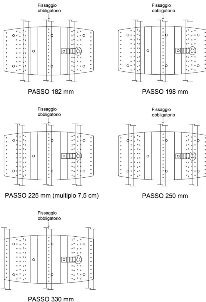
ESEMPI DI CORRETTO FISSAGGIO CON RIVETTI IN RELAZIONE AL PASSO DELLE COSTE DEL SUPPORTO
