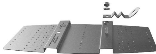
SCHEMA DI ASSEMBLAGGIO
